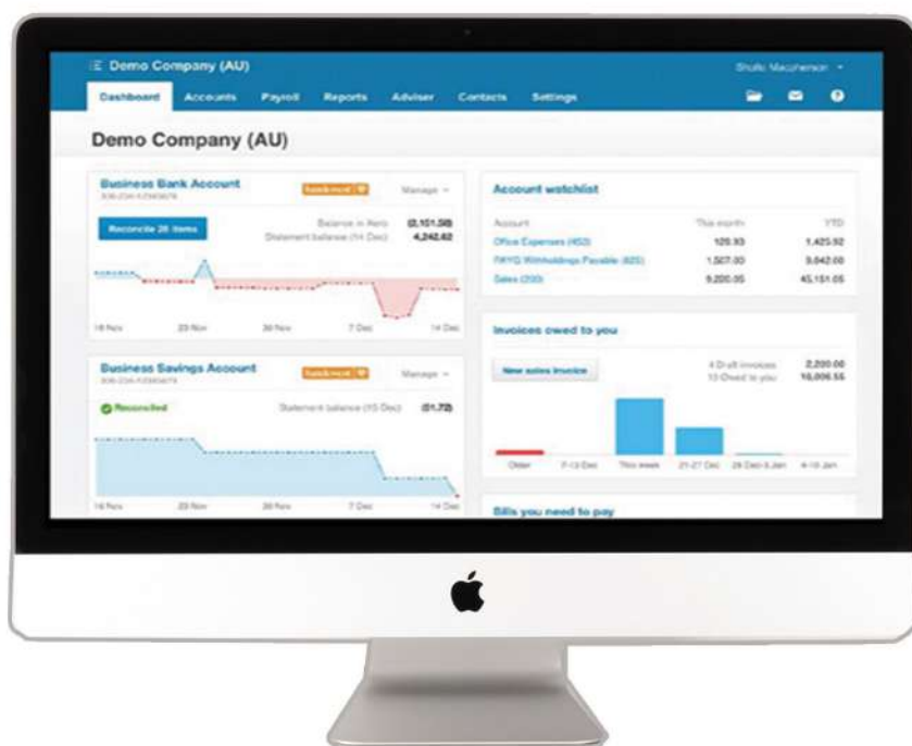
داشبورد - Xero
