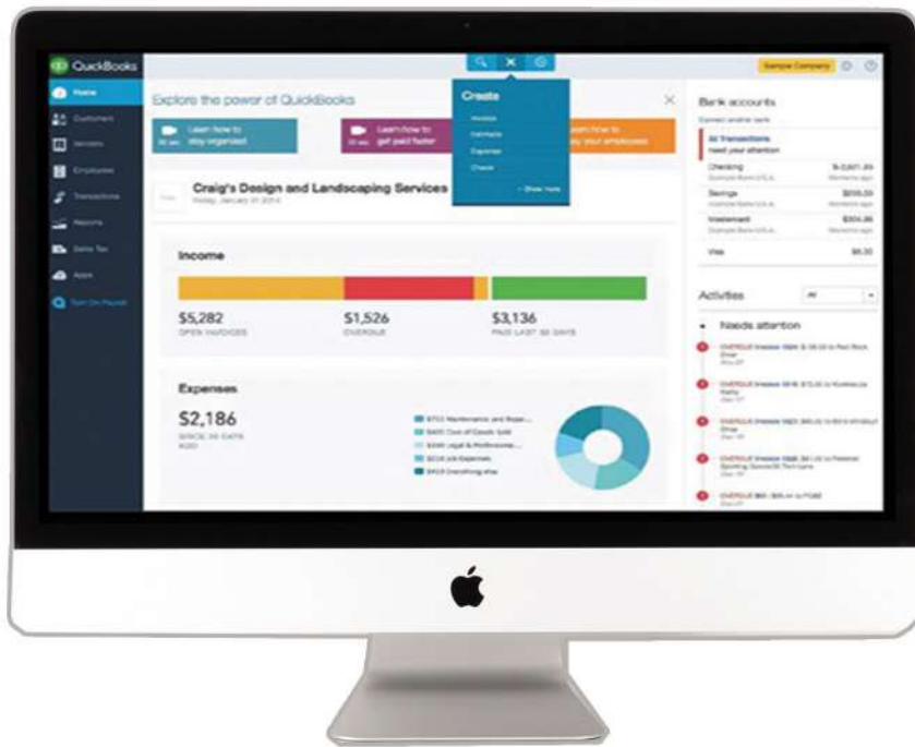
داشبورد Quickbooks
